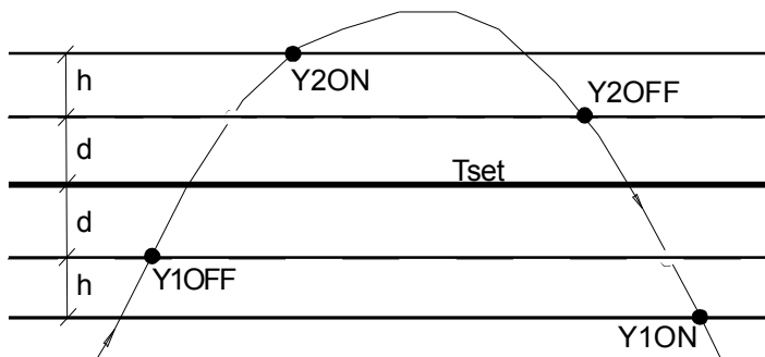
Фиг.1 Времева диаграма на работата на WM-1
