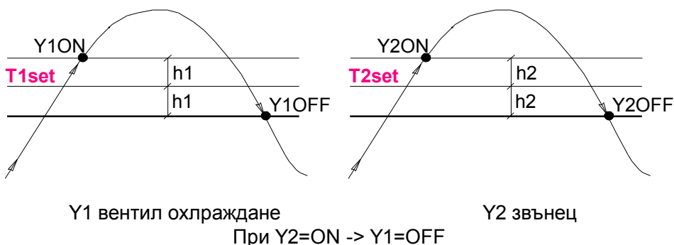
Фиг.1 Времедиаграма на работата на VC3-3RS/Dest
